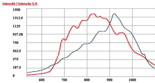
IR Spectrum Circline 1001N
